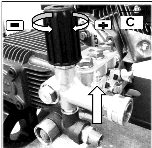
Wersja samozasysająca
